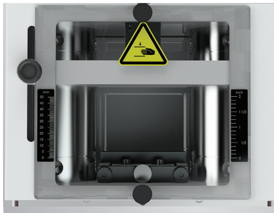
Einstellung der Abisolierlänge Adjustment of the strip length
